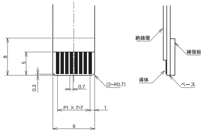
出力部詳細
