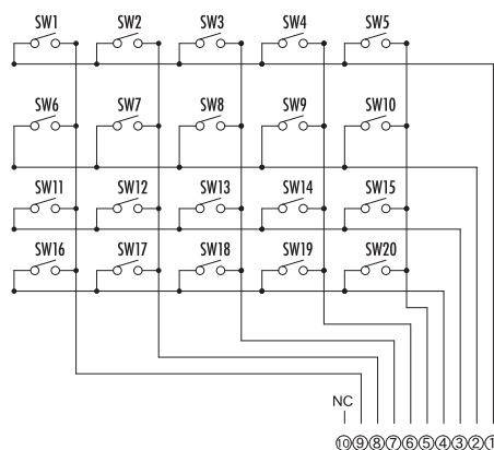
回路図
