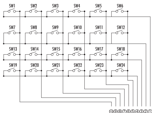
回路図
