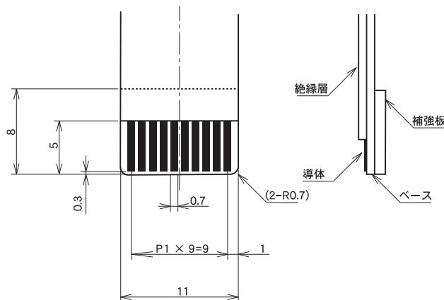
出力部詳細
